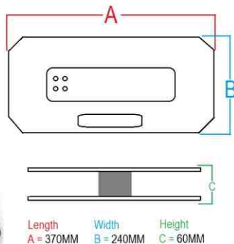
Fig. Pad dimensions
